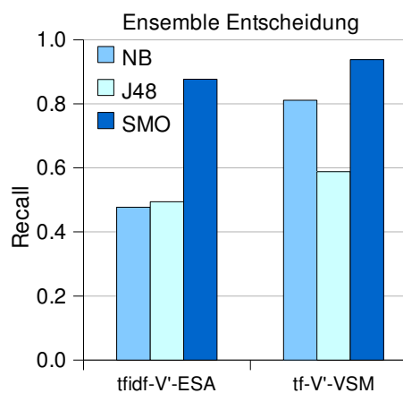
Abbildung 4.2: Ensemble Entscheidung
